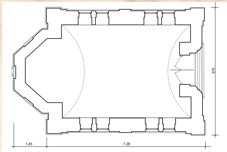
Rzut przyziemia kaplicy
